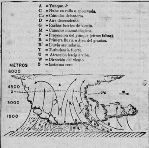
Corte vertical a través de un tipo de tempestad eléctrica térmica
